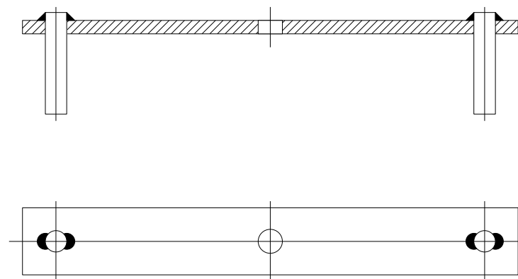
Verrou de montants ech. 1/2
